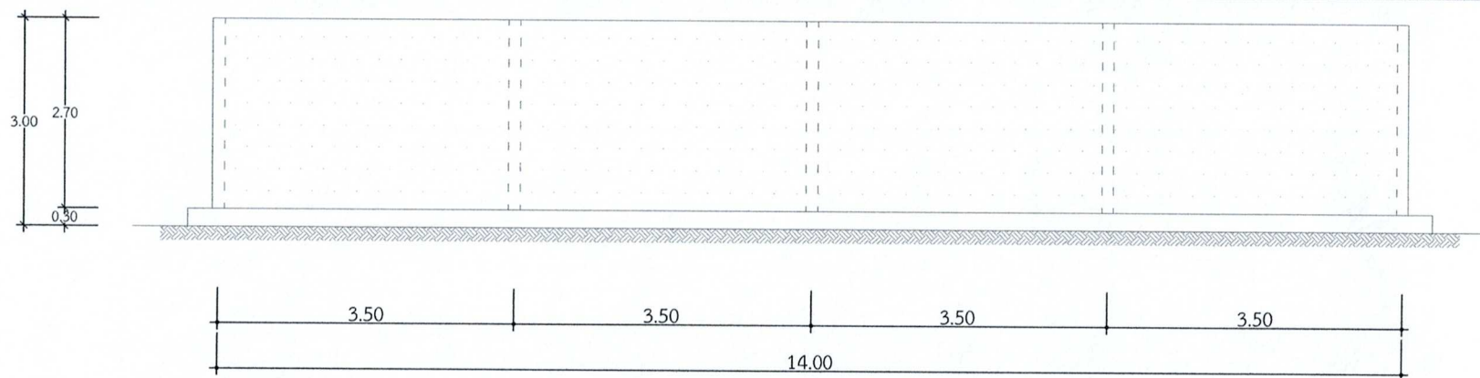
รูปด้านหน้า
