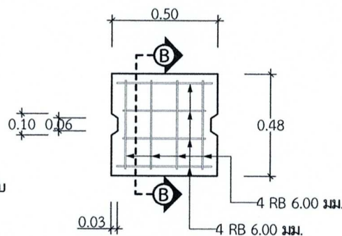
รูปขยายฝารางระบายน้ำ
