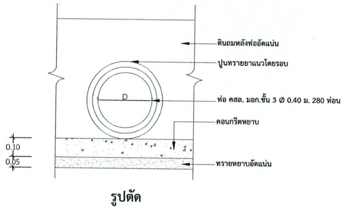
รูปตัด SCALE 1:25
