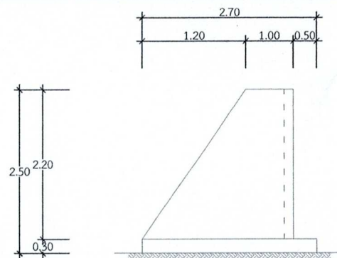
รูปด้านข้าง
