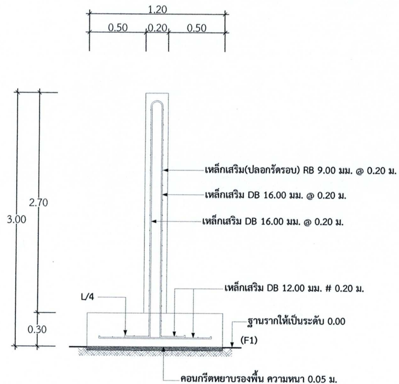
รูปตัด A พร้อมขยายรายละเอียดต่างๆ
