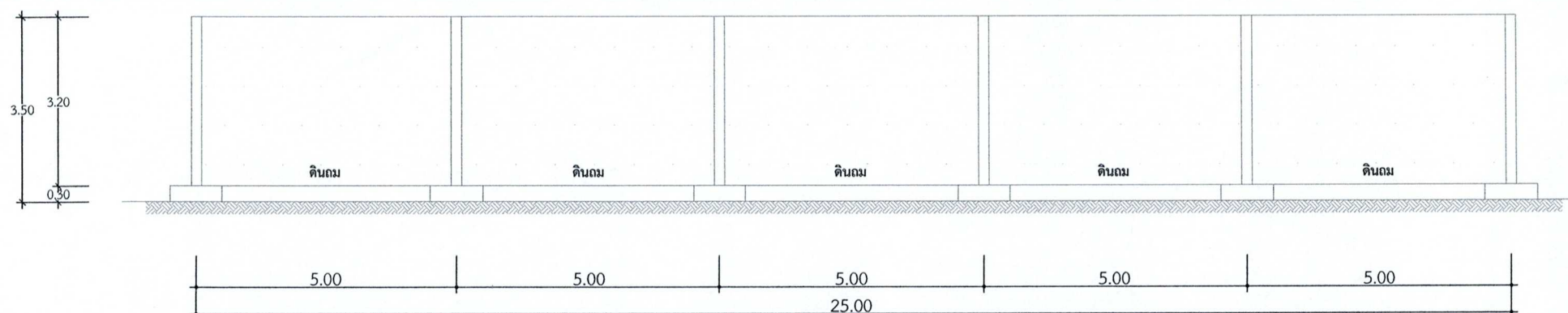
รูปด้านหลัง
