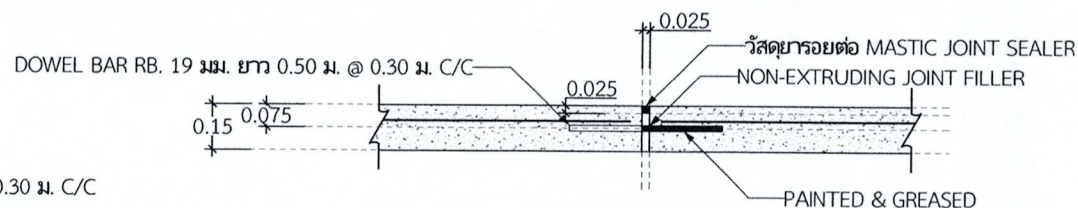
ขยายรอยต่อ EXPANSION JOINT
