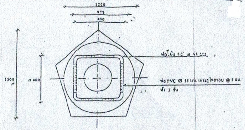
แปลน ชุดเพิ่มระดับอากาศ 1:25
