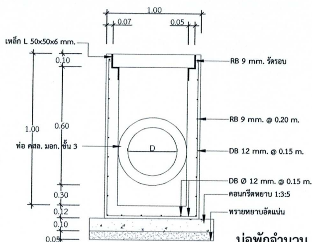
รูปแบบฝาปิดบ่อพัก
