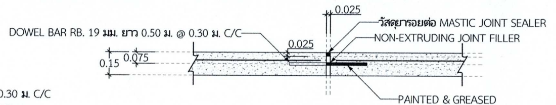
ขยายรอยต่อ EXPANSION JOINT
