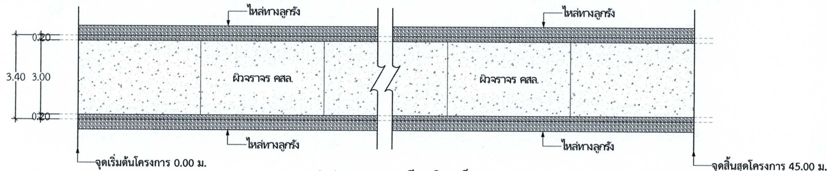
รูปแปลนถนนคอนกรีตเสริมเหล็ก
