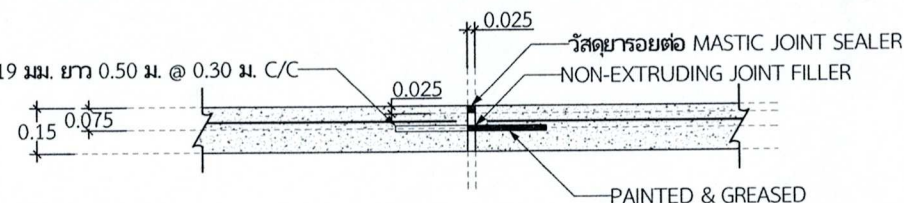
ขยายรอยต่อ EXPANSION JOINT
