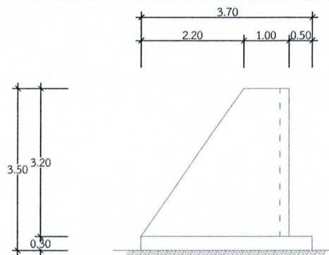
รูปด้านข้าง
