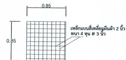
รูปแบบฝาปิดบ่อพัก
