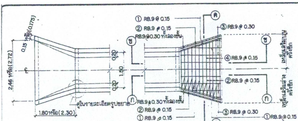
แสดงทรวดทรงแปลนและการเสริมเหล็กขานหน้าและกำแพงปีกหน้าต่อ 1:75
