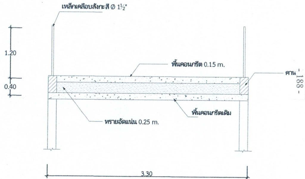
รูปตัดด้านหน้า
