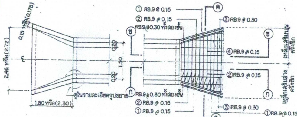
แสดงทรวดทรงแปลนและการเสริมเหล็กขานหน้าและกำแพงปีกหน้าท่อ 1:75
