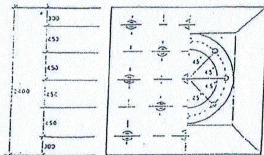
แปลนฐานรากชนิดคอกเข็ม 1:400
