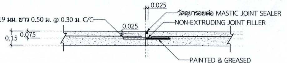
ขยายรอยต่อ EXPANSION JOINT
