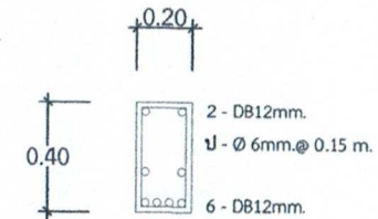
แบบขยายหน้าตัดคาน
