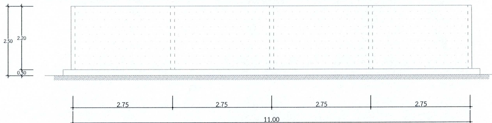
รูปด้านหน้า
