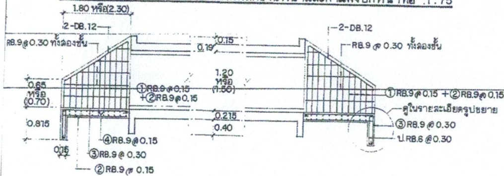
รูปตัด ก - ก 1:75
