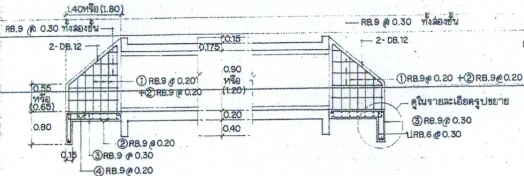
รูปตัด ข - ข 1:75
