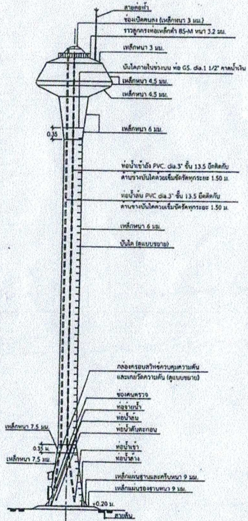
รูปด้านข้างหอถังสูง แบบดังเหล็กรูปทรงถ้วยแฉกเปลว มาตรฐาน 1:100
