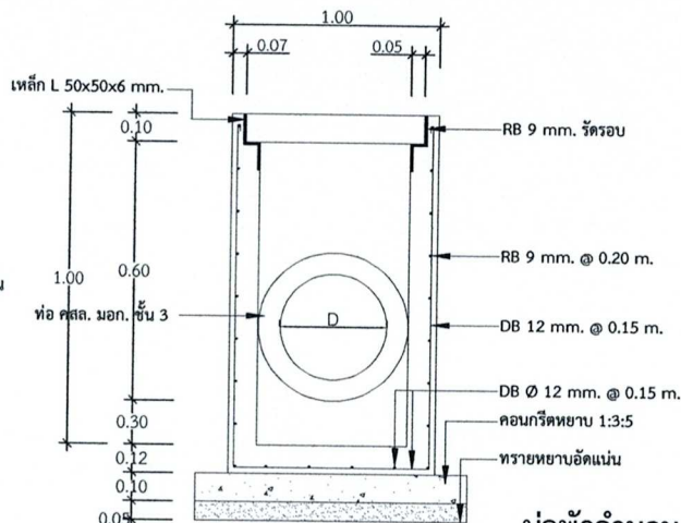
รูปแบบฝาปิดบ่อพัก SCALE 1:25
