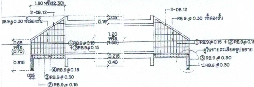
รูปตัด ก - ก 1:75
