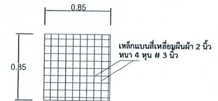
รูปแบบฝาปิดบ่อพัก SCALE 1:25
