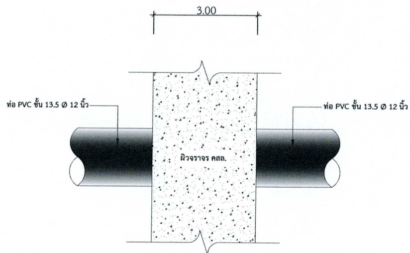
รูปแปลน
