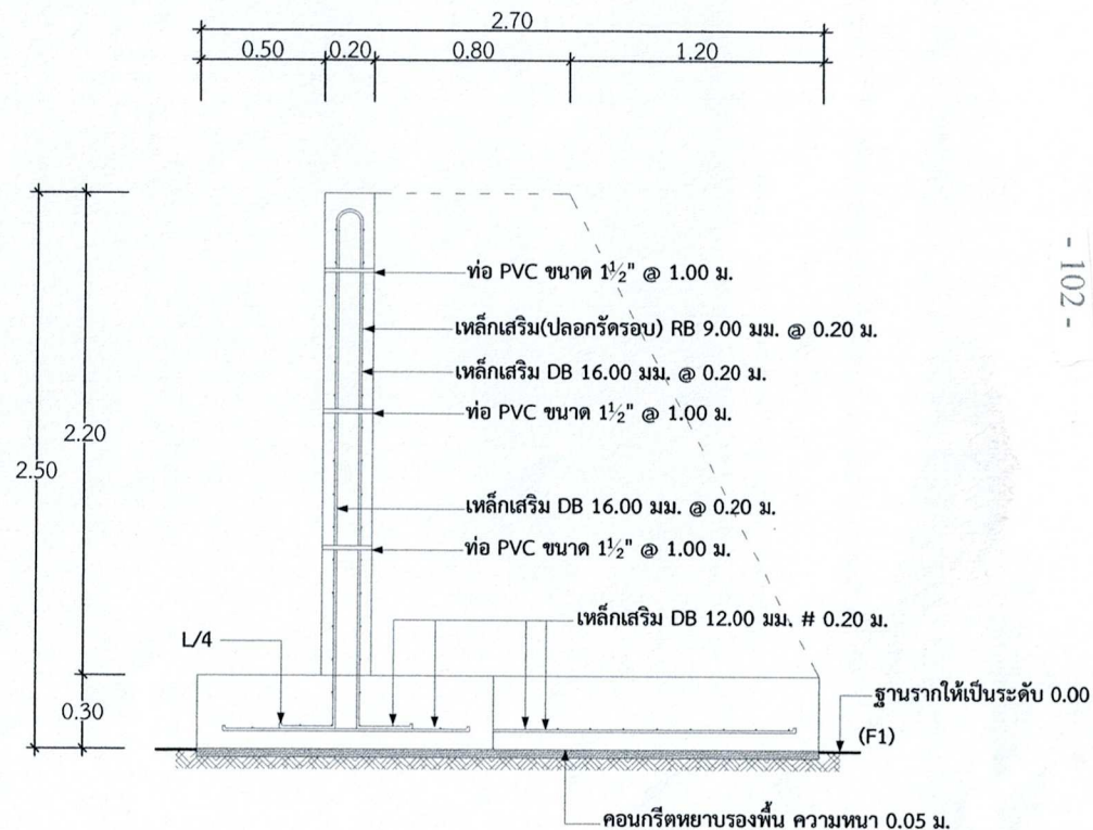
รูปตัด B พร้อมขยายรายละเอียดต่างๆ
