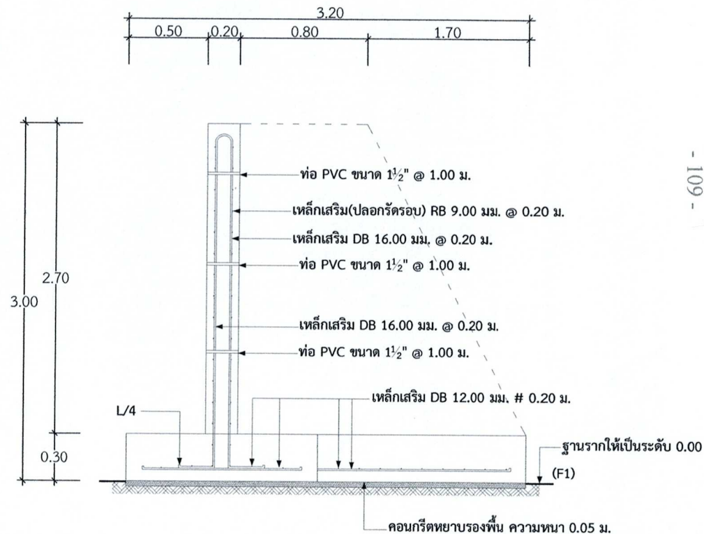
รูปตัด B พร้อมขยายรายละเอียดต่างๆ
