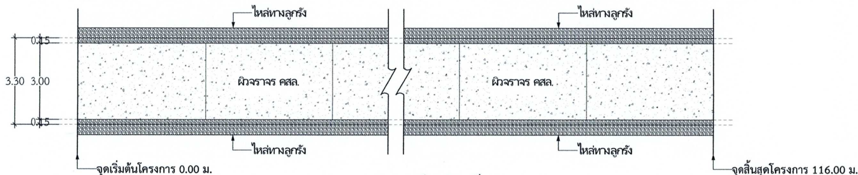
รูปแปลนถนนคอนกรีตเสริมเหล็ก
