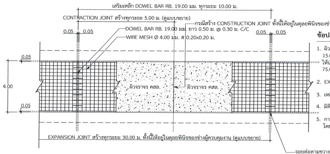
รูปแปลนแสดงการเสริมเหล็กและรายละเอียดต่างๆ
