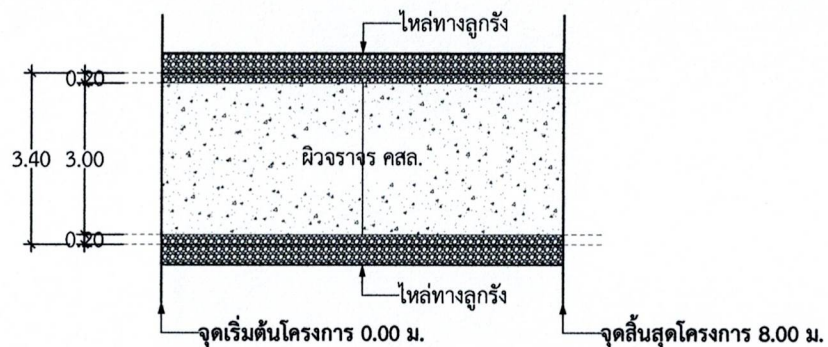
รูปแปลนถนนคอนกรีตเสริมเหล็ก ช่วง 3
