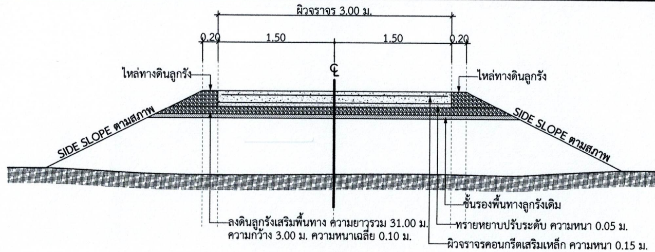
รูปตัดถนนผิวจราจรคอนกรีตเสริมเหล็ก ช่วงที่ 1 - 3
