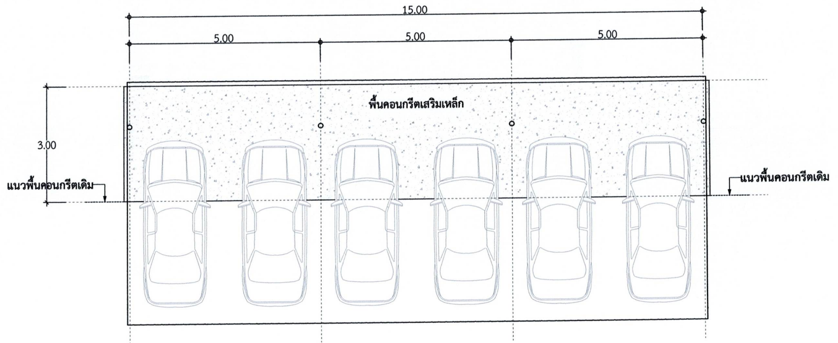
แสดงรูปแบบ SCALE 1:100
