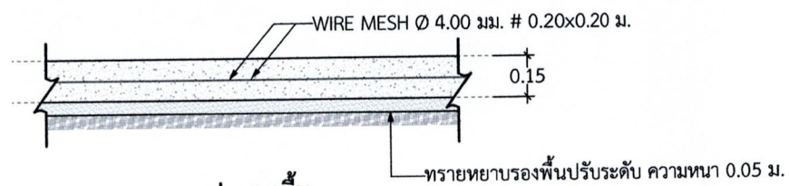
รูปขยายพื้น
