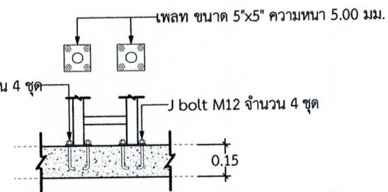
รูปขยายตอม่อ (C1)
