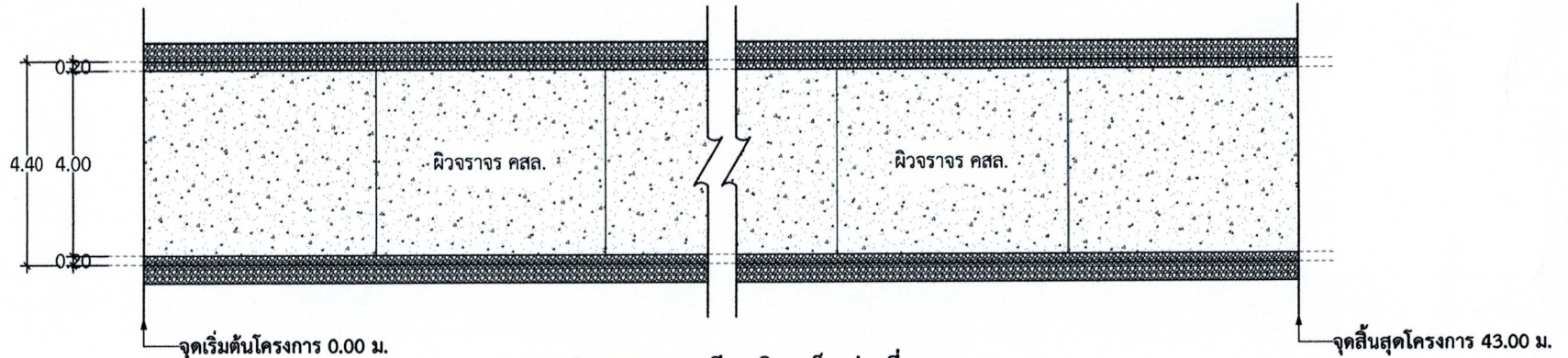
รูปแปลนถนนคอนกรีตเสริมเหล็ก ช่วงที่ 1
