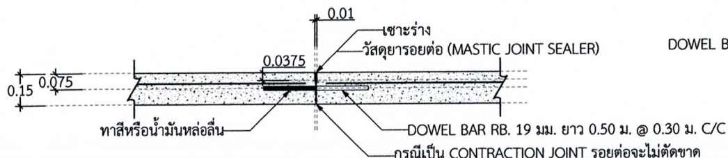
ขยายรอยต่อ CONSTRUCTION JOINT และ CONTRACTION JOINT
