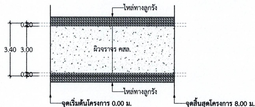
รูปแปลนถนนคอนกรีตเสริมเหล็ก ช่วง 2
