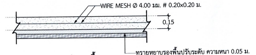
รูปขยายพื้น
