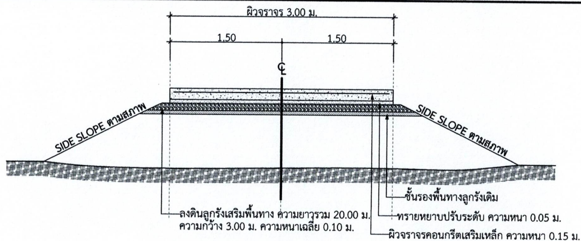
รูปตัดถนนผิวจราจรคอนกรีตเสริมเหล็ก ช่วงที่ 1 - 2
