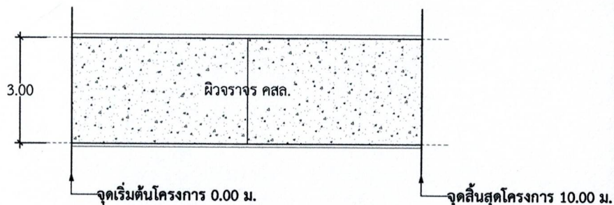
รูปแปลนถนนคอนกรีตเสริมเหล็ก ช่วงที่ 1
