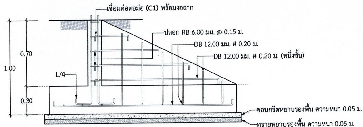
แบบขยายฐานราก F1,C1 พร้อมรายละเอียด
