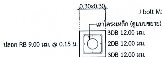
รูปขยายตอม่อ (C1)
