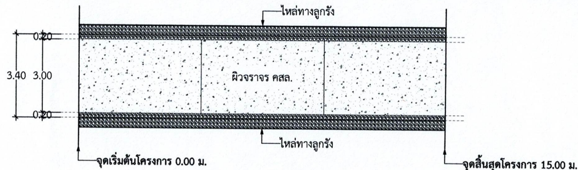
รูปแบบถนนคอนกรีตเสริมเหล็ก ช่วงที่ 1
