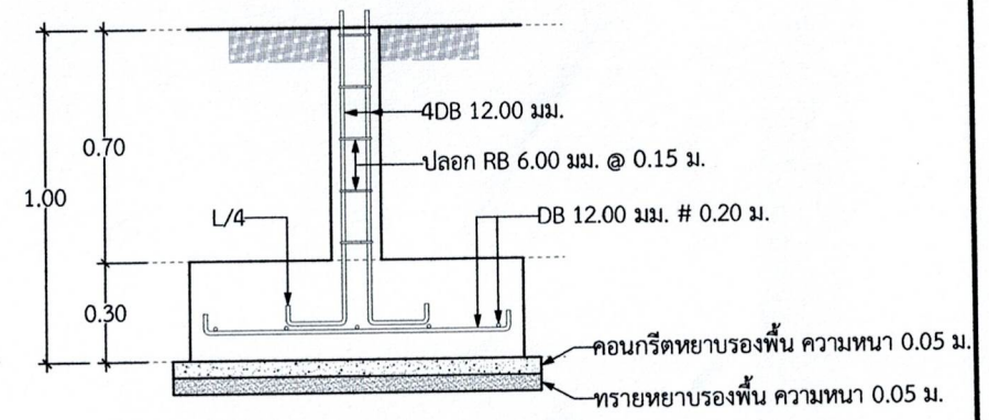
แบบขยายฐานราก F2,C2 พร้อมรายละเอียด
