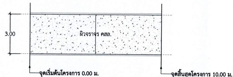
รูปแปลนถนนคอนกรีตเสริมเหล็ก ช่วงที่ 2
