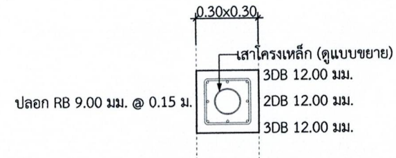
รูปขยายตอม่อ (C1)
