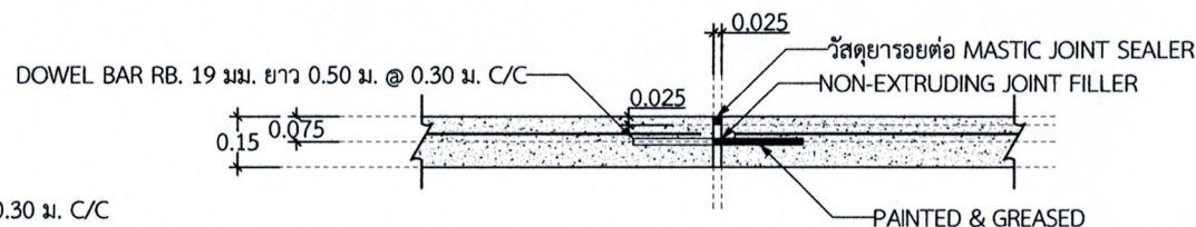
ขยายรอยต่อ EXPANSION JOINT
